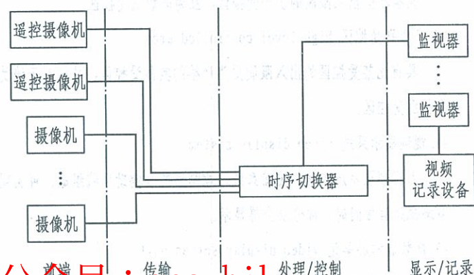
时序切换模式
