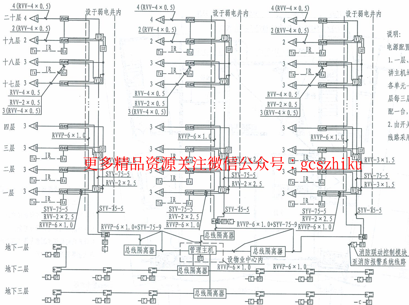
可视对讲系统方案二
