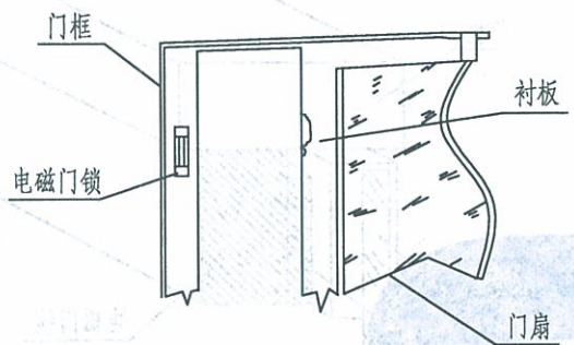
(a) 安装示意图
