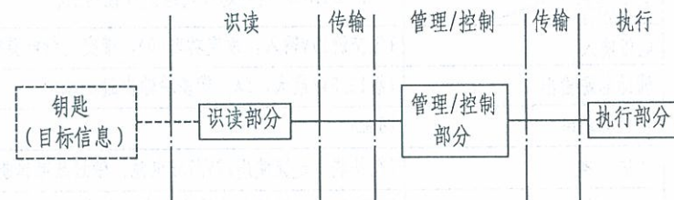
(b) 分体型结构组成之二
