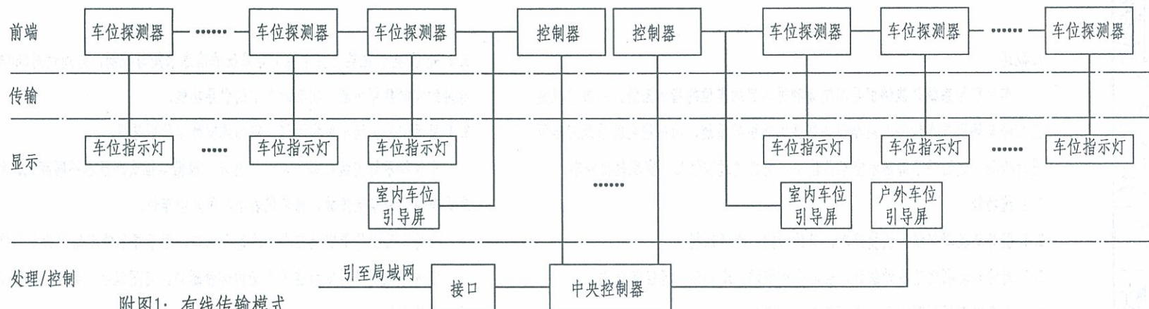
附图1: 有线传输模式
