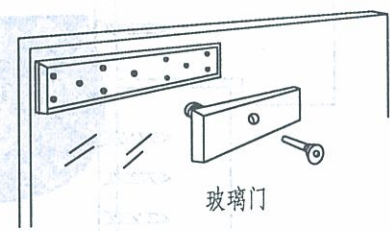
(c) 衬板安装示意图(二)
