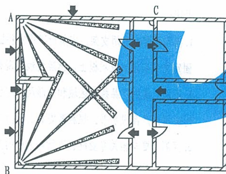
2. 被动红外探测器的布置示例
